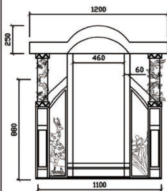
正立面
