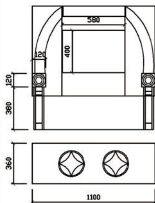
平面图
