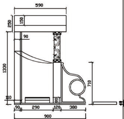
側立面
